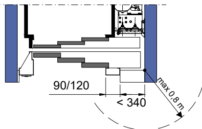
PIANTA PIANO GRUPPO DI MANOVRA TELAIO PORTE MRF 90/120 (STANDARD ED EI120)
