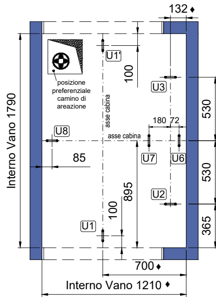
GANCI IN TESTATA (a cura del Cliente)
