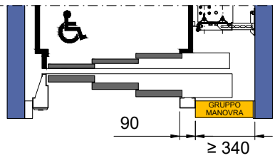
PIANTA PIANO GRUPPO DI MANOVRA TELAIO PORTE MRF 90 (STANDARD ED EI120)
