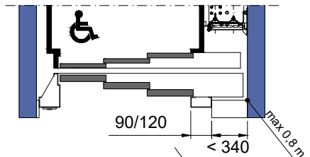
PIANTA PIANO GRUPPO DI MANOVRA TELAIO PORTE MRF 90/120 (STANDARD ED EI120)
