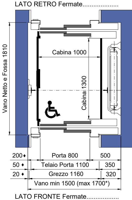
PIANTA VANO CORSA TELAIO PORTE NF (EI120)
